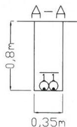
1 - Trubka KOPOFLEX 110
