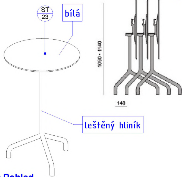
3D Pohled
