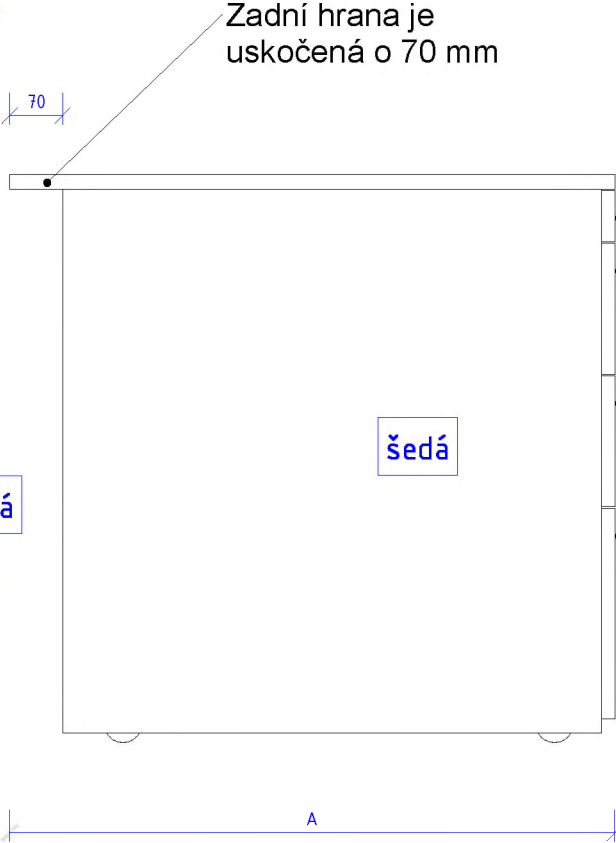
Pohled boční 1 : 10
