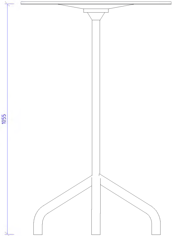
Pohled čelní 1 : 10
