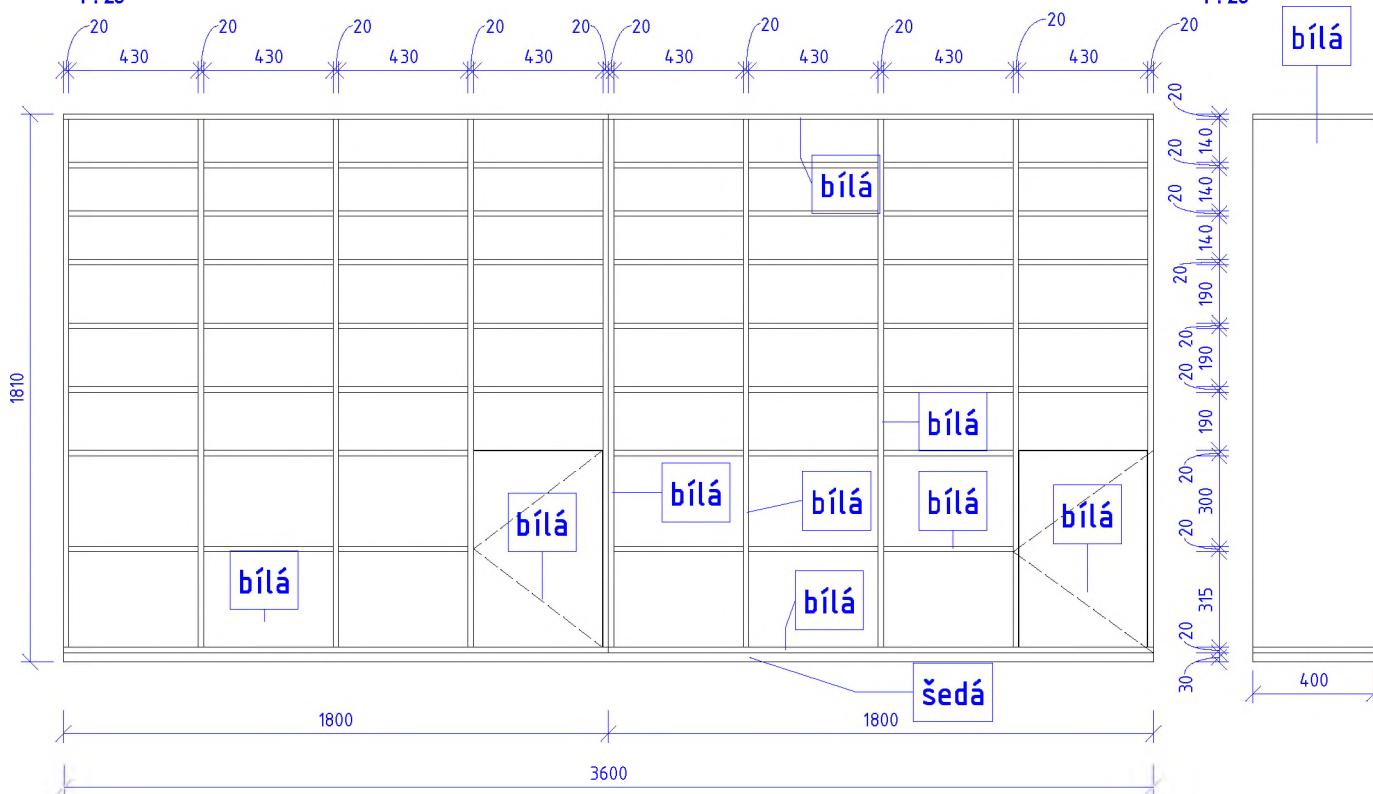
Pohled čelní
