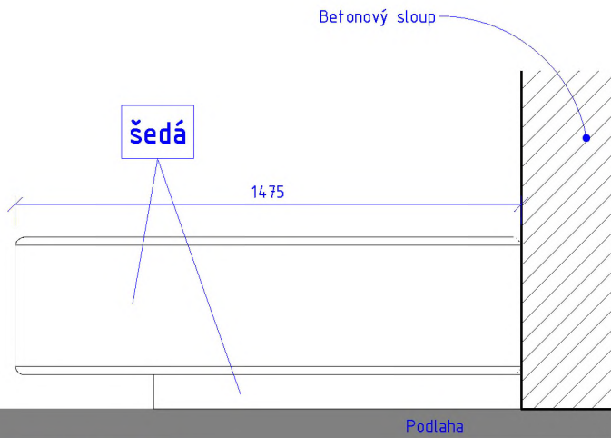
Pohled boční 1 : 20
