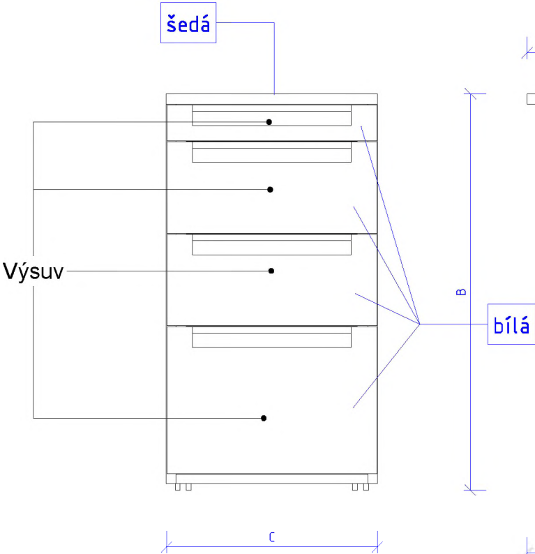
Pohled čelní 1 : 10
