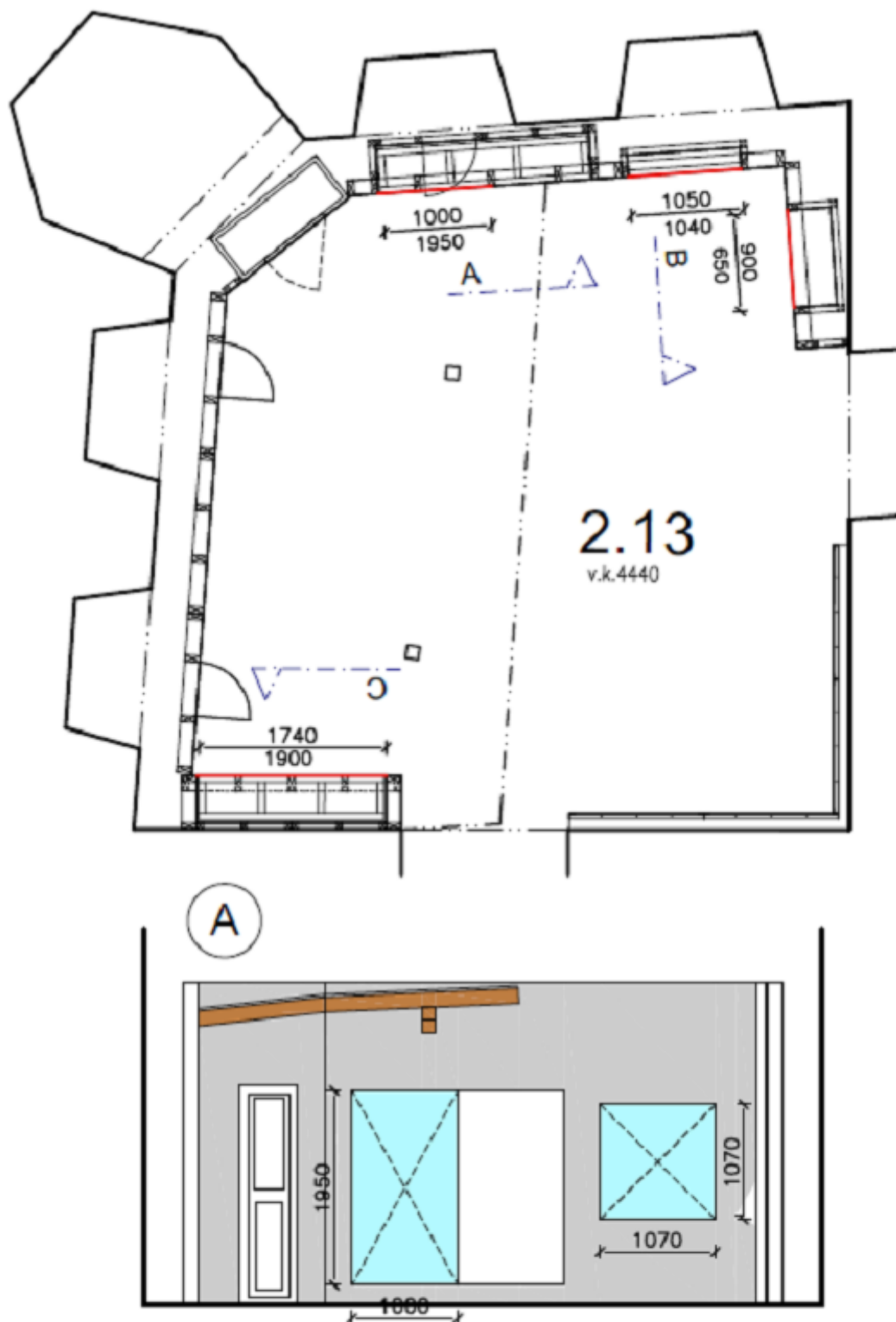
příloha č. 1 ke smlouvě o dílo Schematický náčrt s označením předmětu výměny zasklení
