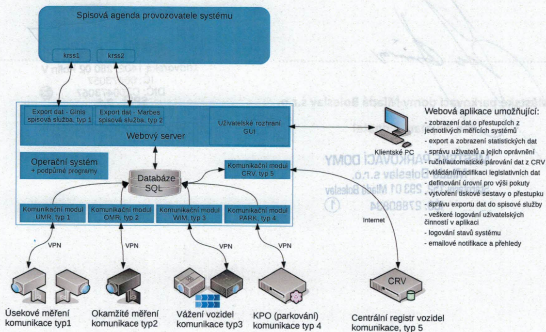
Komunikační schéma nadstavbového systému správy přestupků
