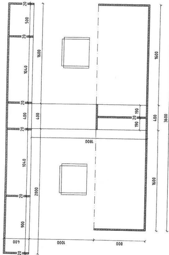
PŮDORYS PRACOVNÍHO MÍSTA
