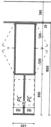
PŮDORYS STŘEDNÍ SKŘÍŇKY
