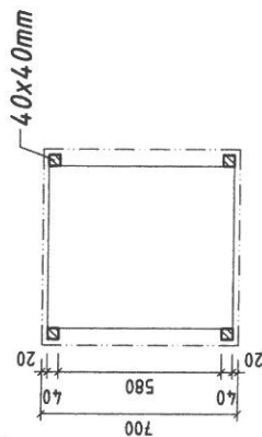
PŮDORYS
