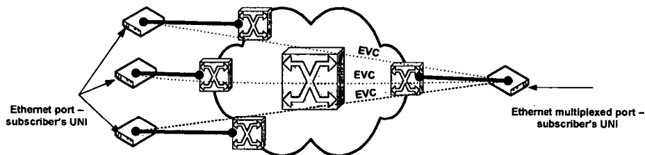
Obr. 2 - Schéma varianty Služby v konfiguraci „Bod – Multibod“
