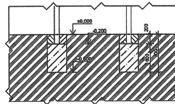
ŘEZ TRÁVA
