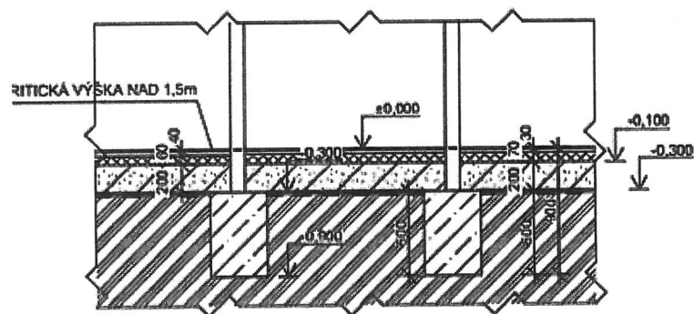
ŘEZ EPDM
