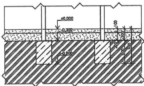
ŘEZ KAČÍREK
