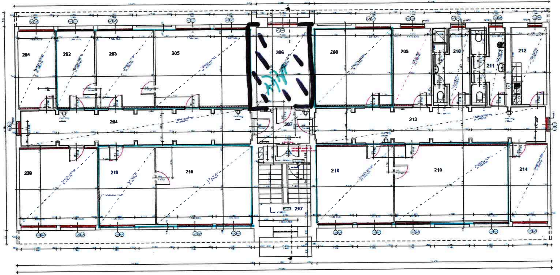
Půdorys 2.NP - nový stav, M 1:50
