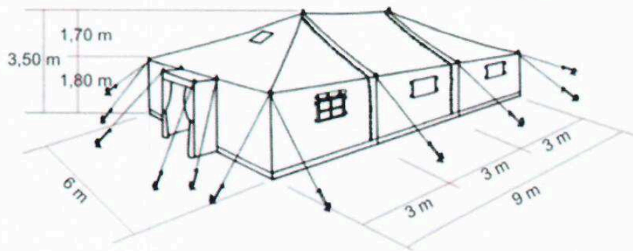
Výkresová dokumentace - rozměry předních, nástavných a zadních dílů S 65
