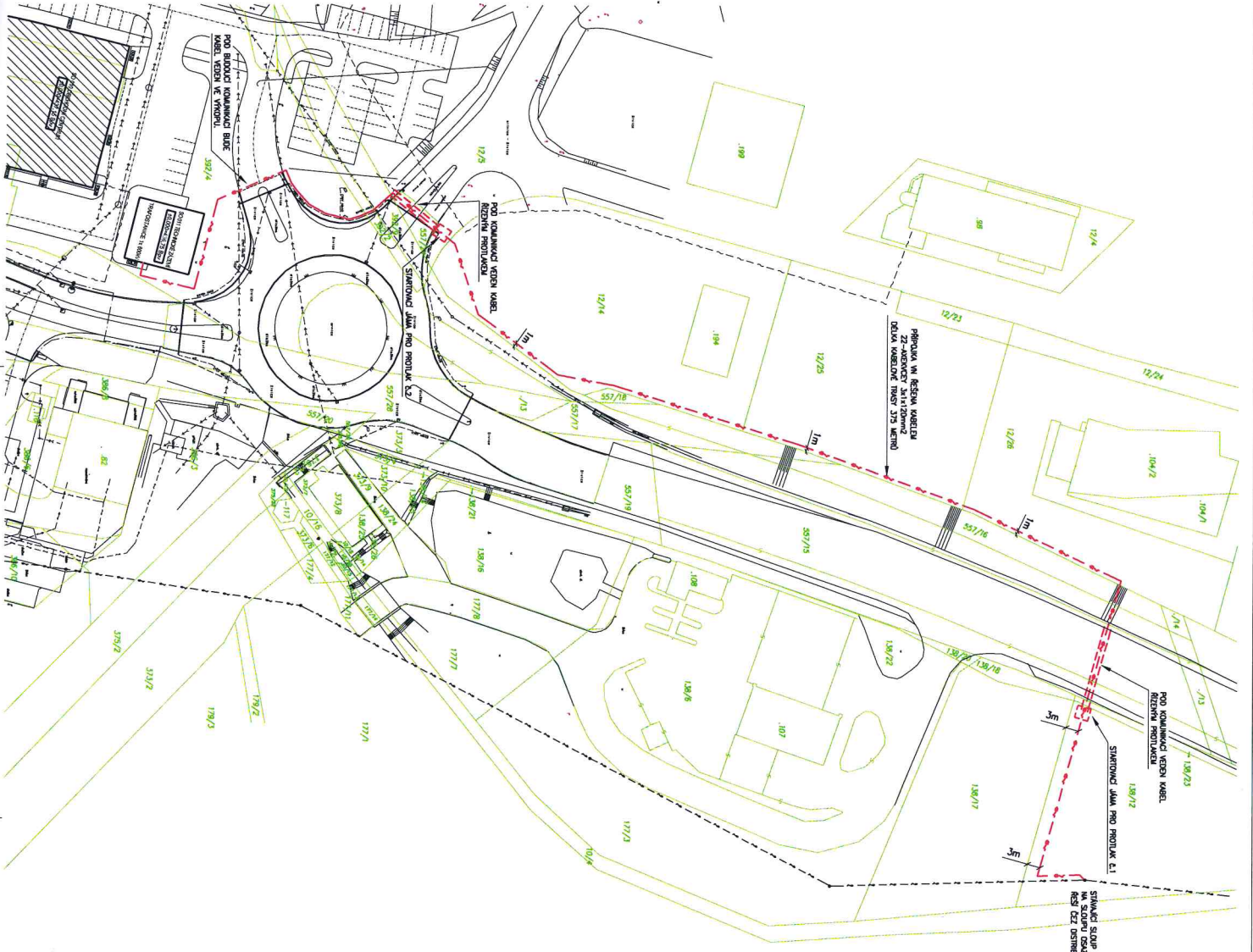
ÚZDENÍ KABELU VE VODNÍM TERÉNU
