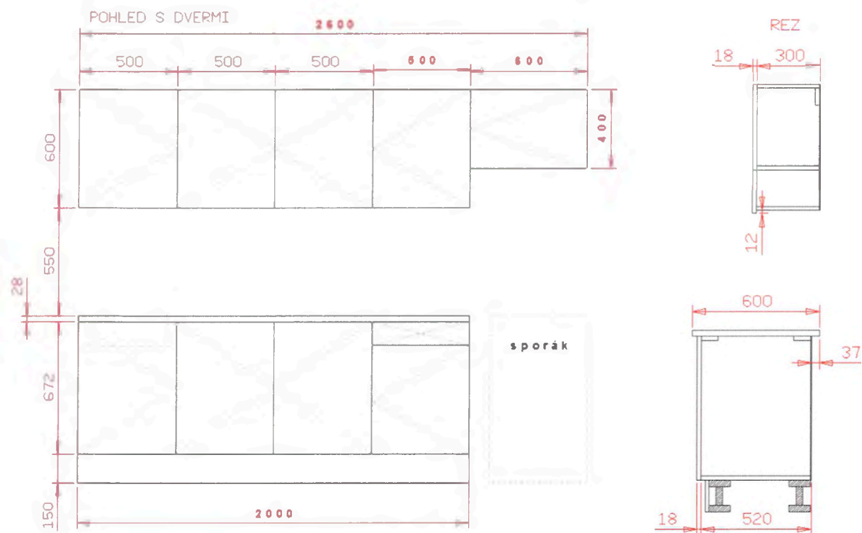
Obr. 2 Typová kuchyně TYP 2, pohled a řez
