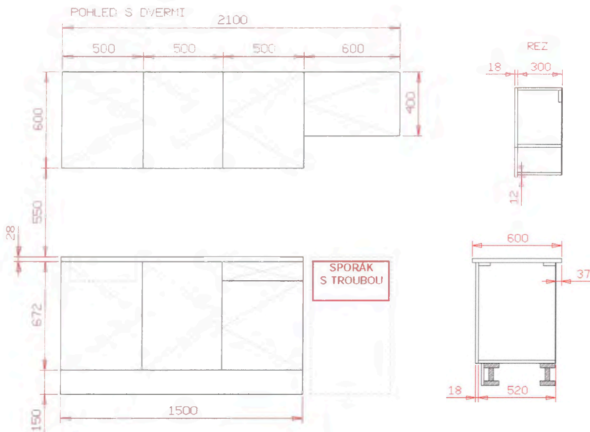
Obr. 1 Typová kuchyně TYP 1, pohled a řez
