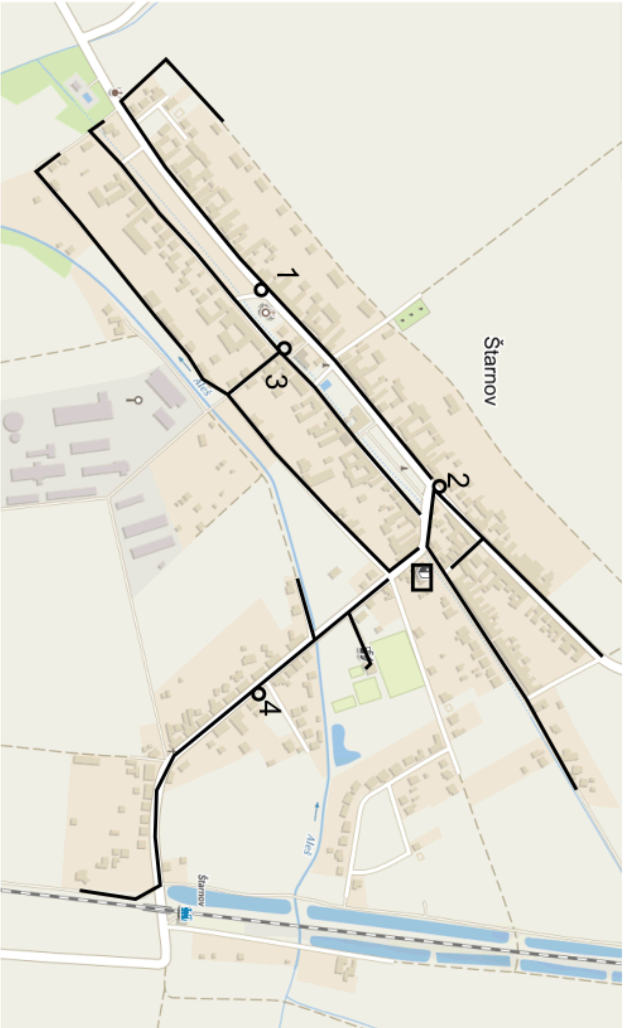
Obr. 1 - mikrotrubičky HDPE 7/3.5 od rozvaděčů ke klientům
