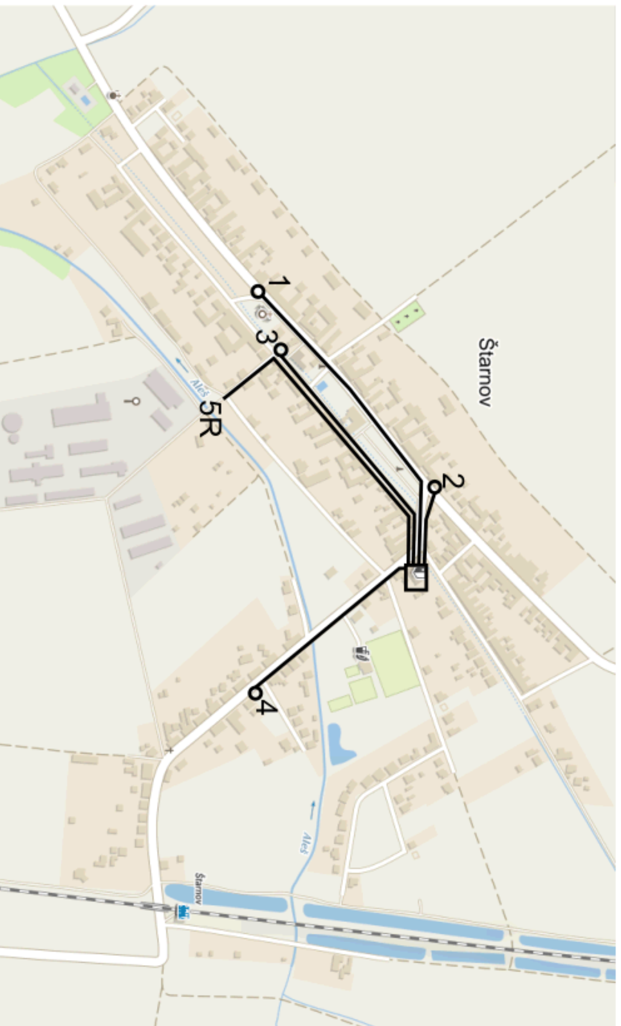
Obr.2 - mikrotrubičky HDPE 12/8 z CentralOffice do rozvaděčů
