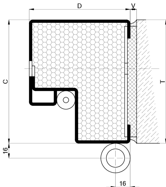
DETAIL ZÁRUBNĚ
