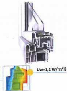
Dvojité zasklení 24 mm Hliníkový distanční rámeček
