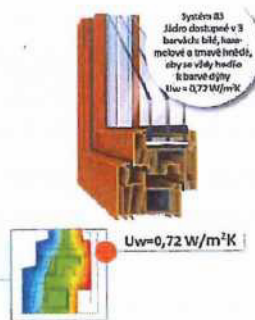
Trojité prosklení 48 mm Distanční rámeček SWISSPACER V, argon
