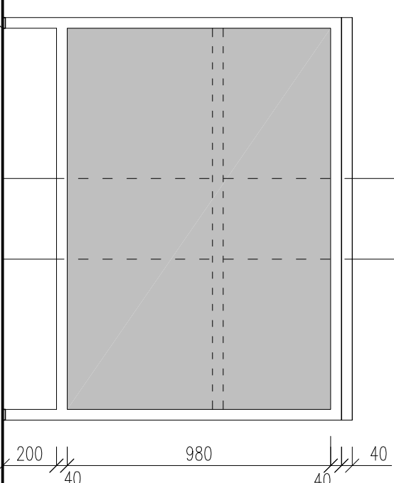
POHLED BOČNÍ
