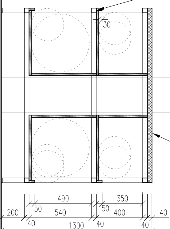
PŘÍČNÝ ŘEZ
