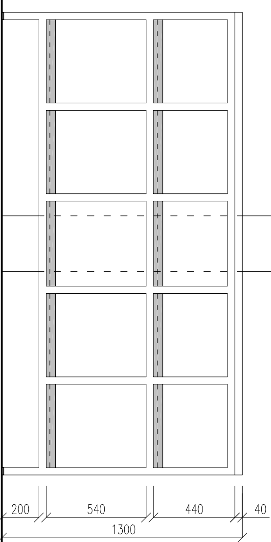
POHLED ČELNÍ
