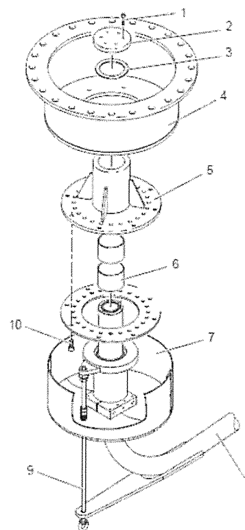
Technický náčrt
