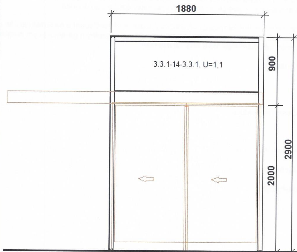
Použití sensorů v průchodu dle ČSN EN 16005 – pohled exteriér
