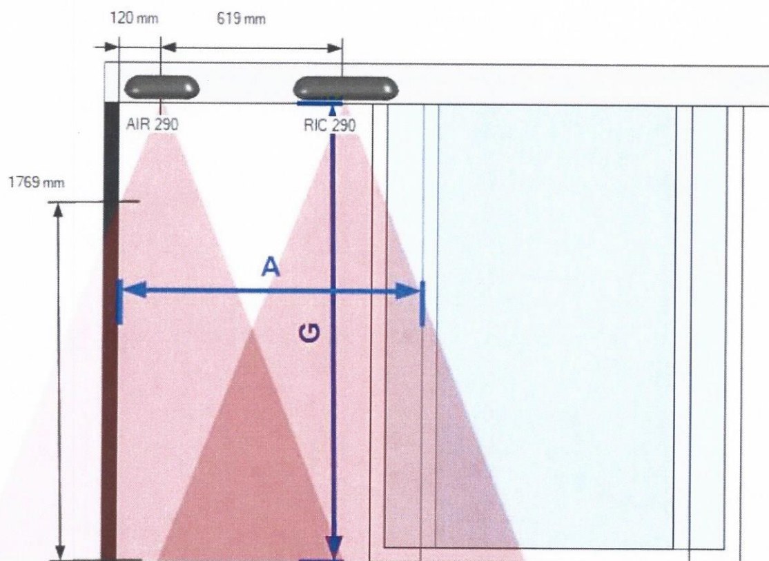
Použití sensorů v průchodu dle ČSN EN 16005 – pohled exteriér
