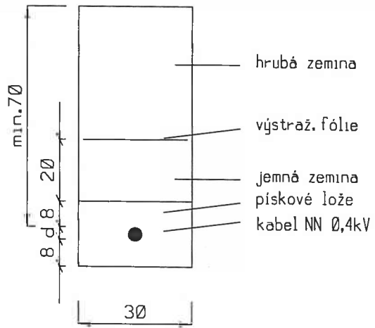
Řezy uložení kabelu v zemi
