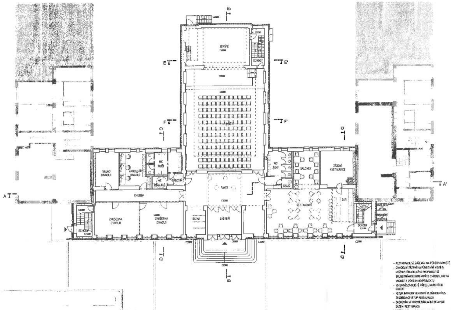
DIVADLO SOLIDARITA 2019_02_06 PŮDORYS 1.NP
