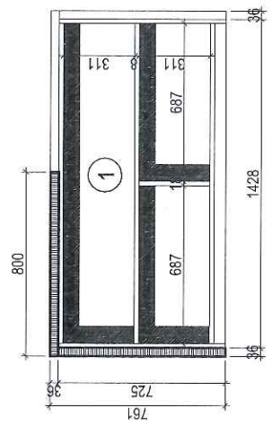
ŘEZ NÁBYTKEM A-A
