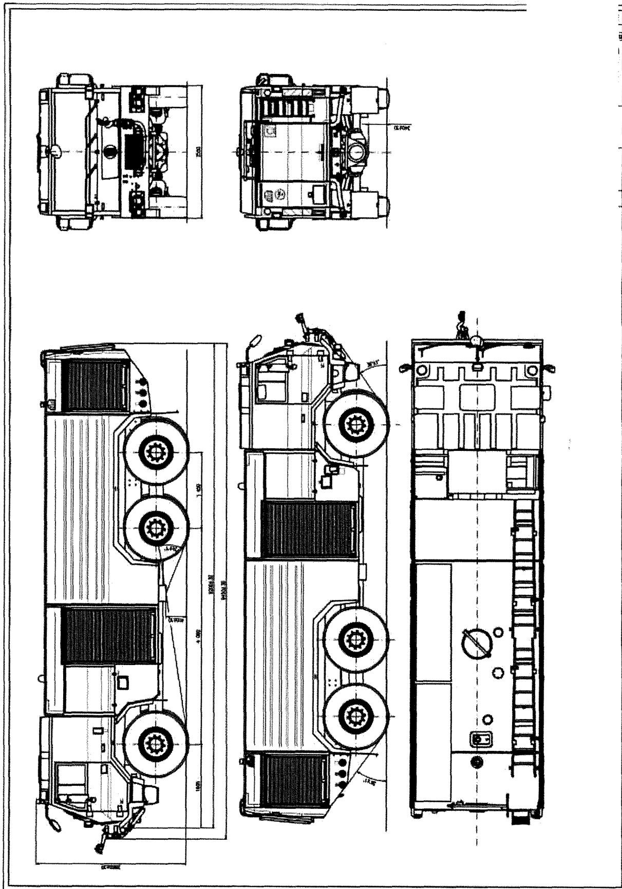
Přílohy: Rozměrový výkres vozidla
