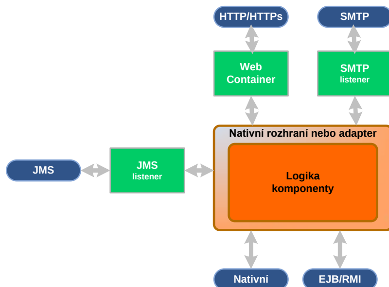
Obrázek 1.3-5: Obecné schéma komponenty
