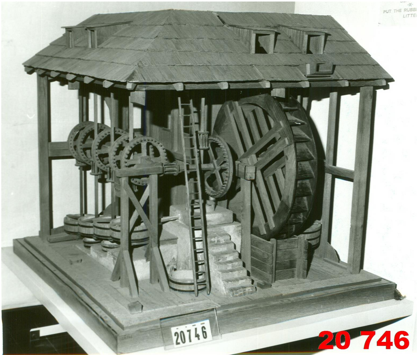
Inventární číslo 20746 – Model jílovské úpravny na zlatou rudu
