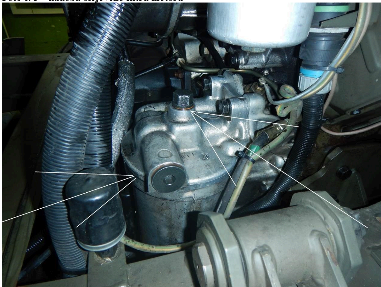
Foto č. 5 – nádoba olejového filtru motoru
