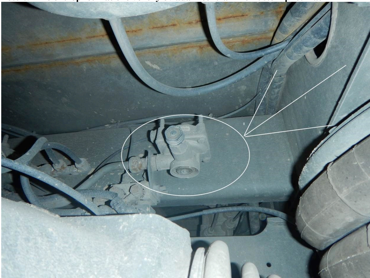
Foto č. 4 – elektropneumatické ventily ovládání centrálního huštění pneumatik
