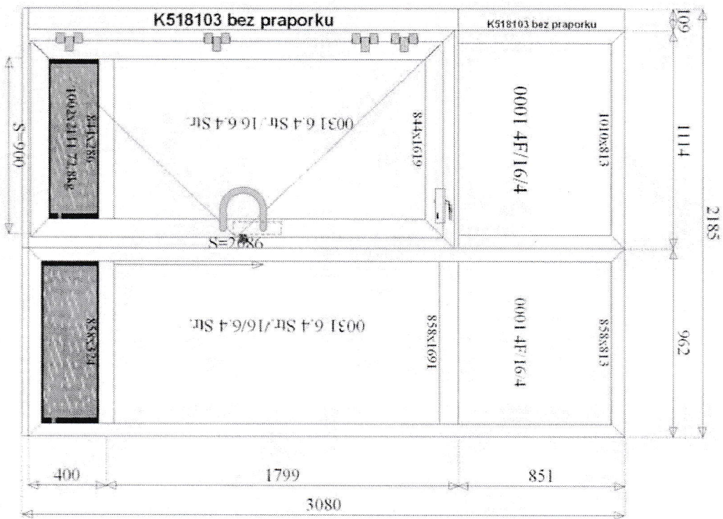
STATICKÉ PROFILY - ZE VNITŘÍ!!!
