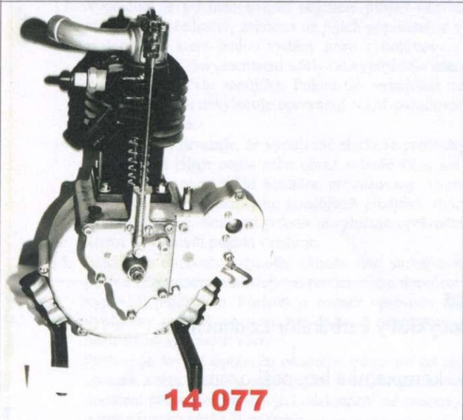
14077 Motocyklový motor Orion 2,75 ks
