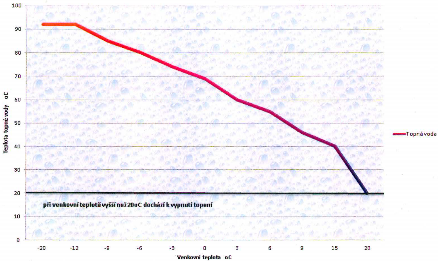
Příloha č. 1 - Regulační křivka
