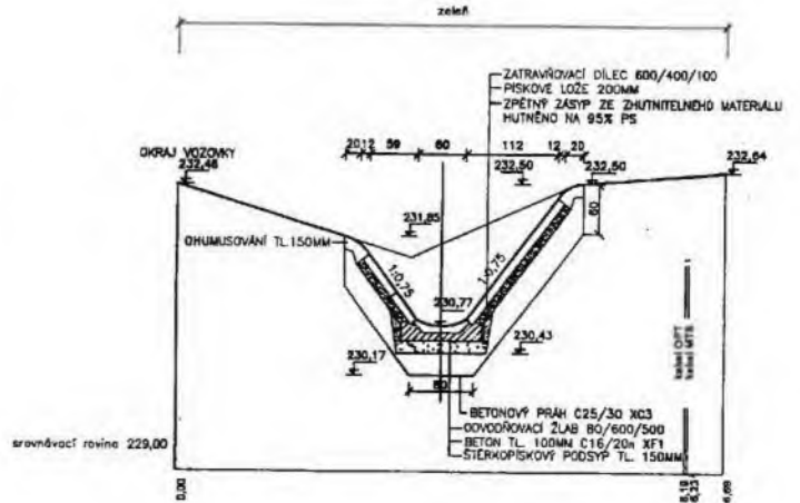
ŘEZ 3-3' 52,82m
