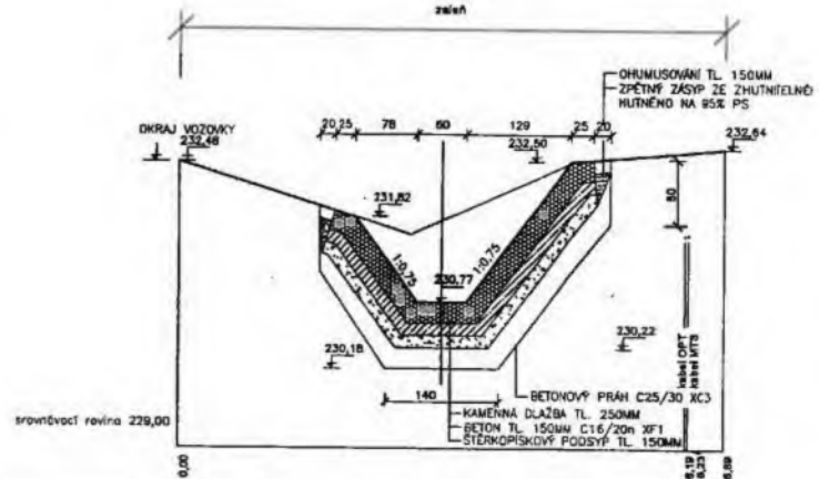
ŘEZ 4-4' 53,12m
