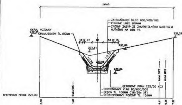
ŘEZ 2-2' 26,46m
