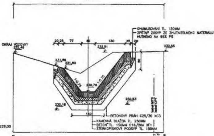
ŘEZ 6-6'
