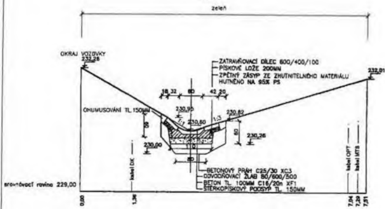
ŘEZ 1-1' 0,3m
