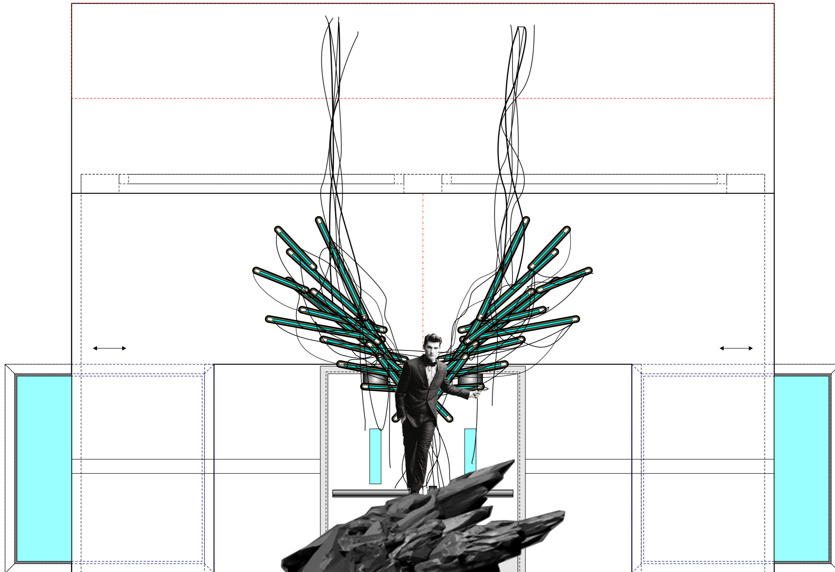
ANGEL WINGS m1:25 trubice LED 1200 - 10ks / 900 - 6ks / 600 - 14ks kabely věšeno tah - sklopný mechanismus
