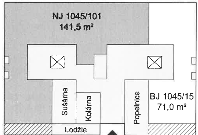
3.NP
