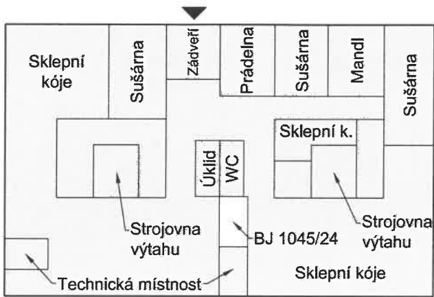
1.PP
