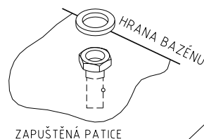
ZAPUŠTĚNÁ PATICE
