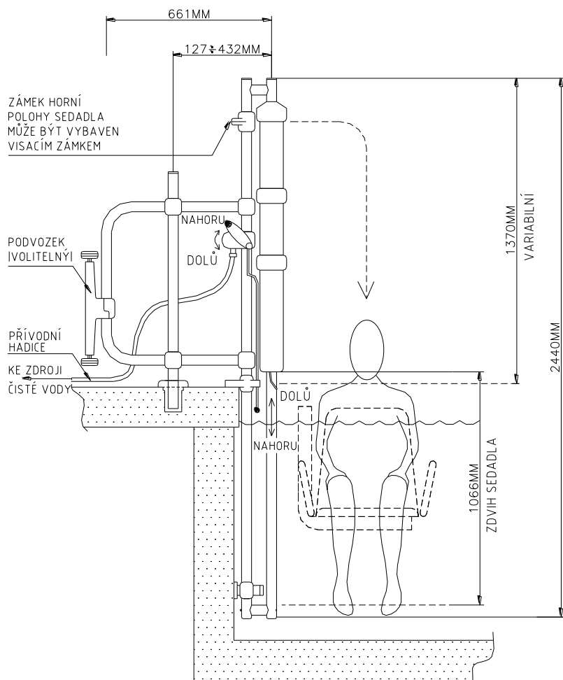
PATICE NA PODLAHU
