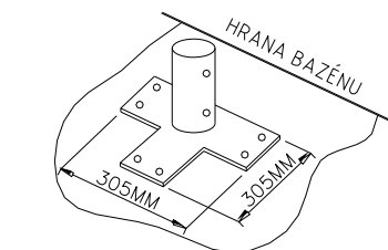
PATICE NA PODLAHU
