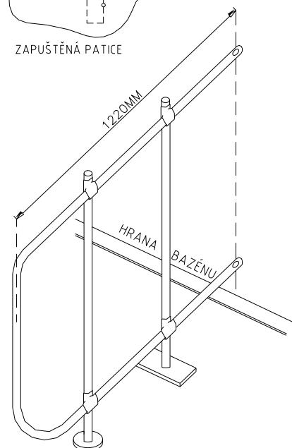
DVOJITÁ PODPĚRA S PRODLOUŽENOU "C" TRUBKOU IPOUZE NA ZVLÁŠTNÍ OBJEDNÁVKUI
