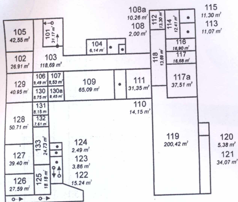
PŘÍZEMÍ (1.NP)
