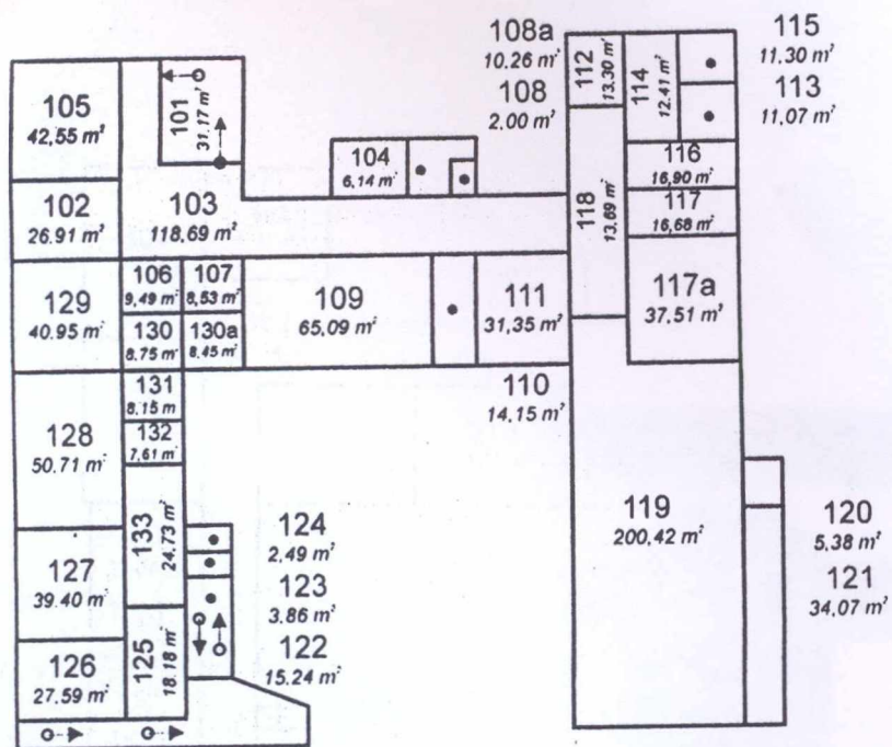
PŘÍZEMÍ (1.NP)
