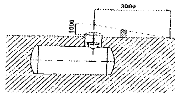
Ochranný prostor podzemního zásobníku
