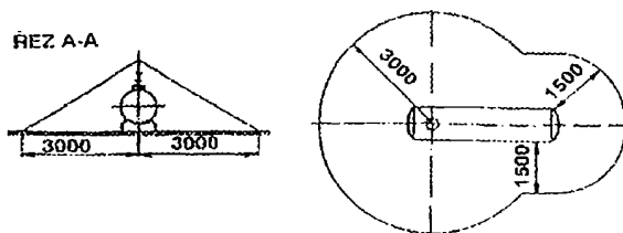
Ochranný prostor ležatého nadzemního zásobníku
