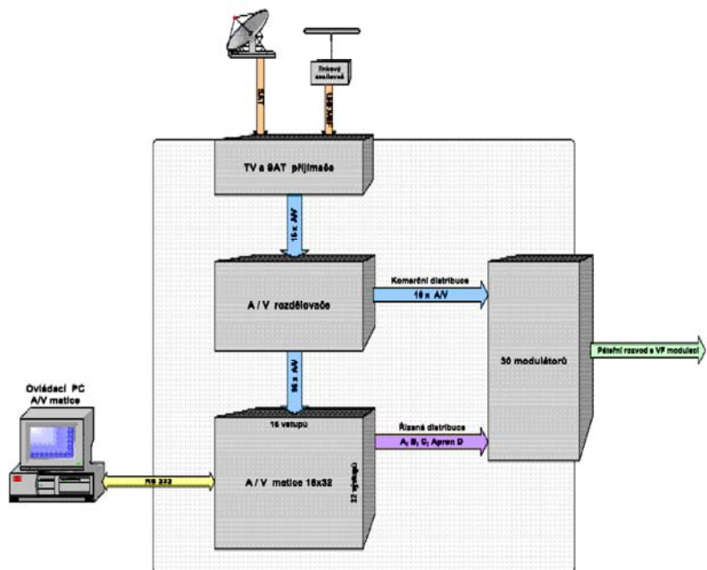
Blokové schéma AV matice 16 x 32 - současný stav
