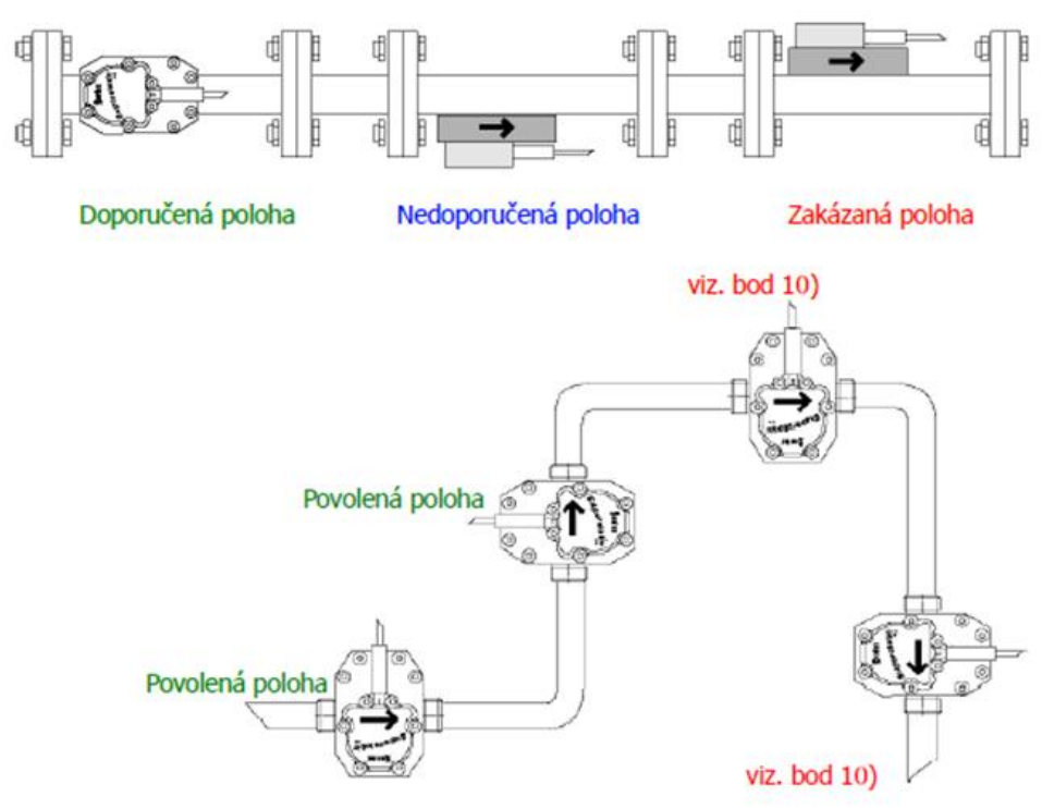
Schéma montáže průtokoměru (obrázek č. 3)
