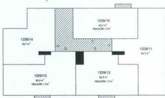
3.NP – 2.PATRO
