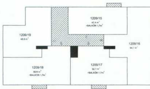
4.NP – 3.PATRO
