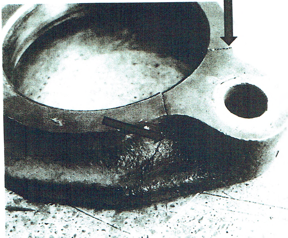
Obr.č.6 – detail praskliny na unašeči náhonu tělesa ventilátoru chlazení motoru
