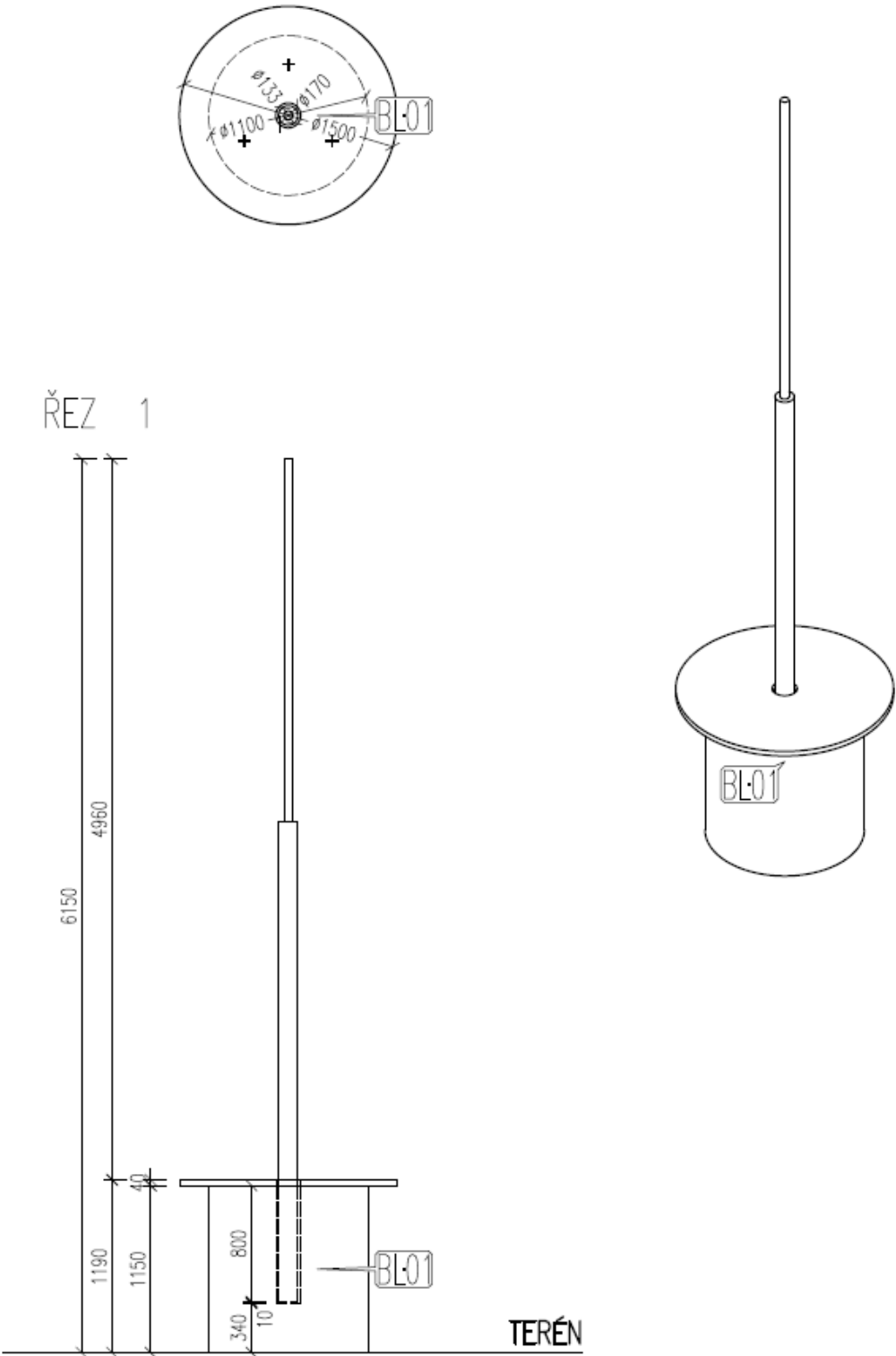
Příloha č. 1 Výkres mobilního betonového bloku se stožárem
