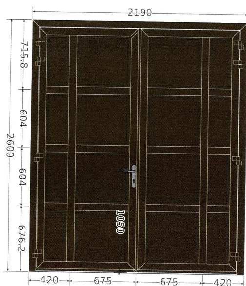
Vnitřní pohled
