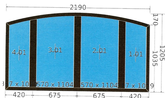
Vnitřní pohled
