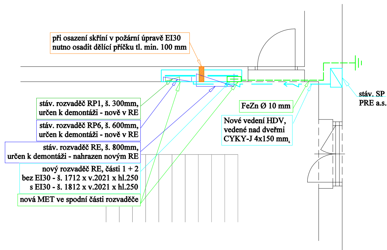
osazení stávajících rozvaděčů v prostoru schodišťové chodby
