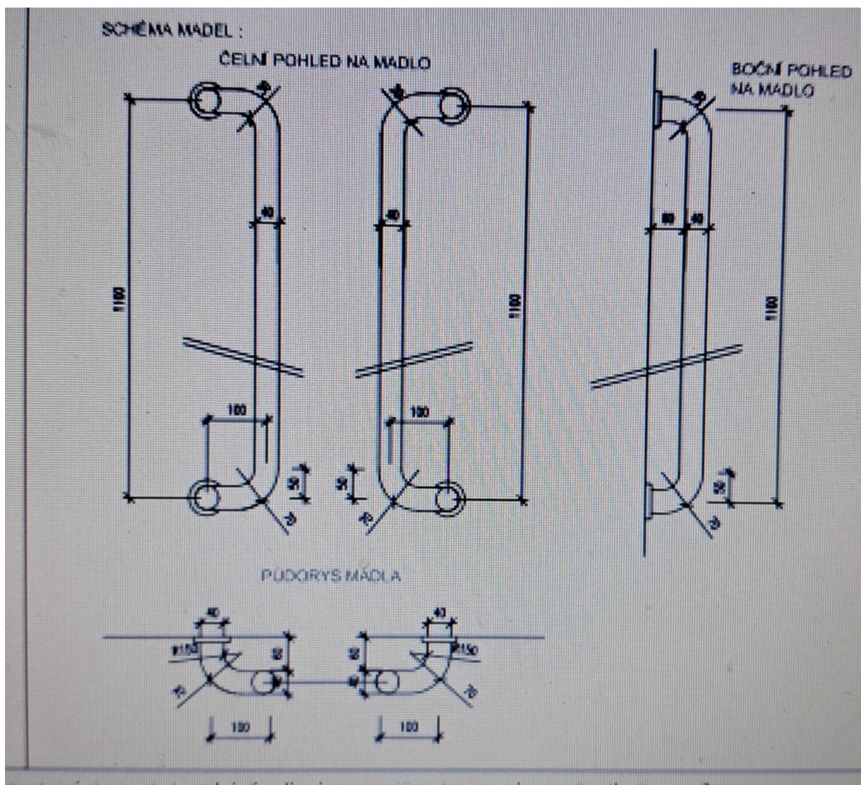
Výrobní výkres madla z dokumentace pro rekonstrukci kina.
