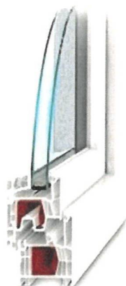
Okno CLASSIC 76 - 6 komorový profil 76mm s izolačním dvojsklem U_g = 1,1 \text{ W.m-2.K-1} Celkové U_w \leq 1,1 \text{ W.m-2.K-1}
