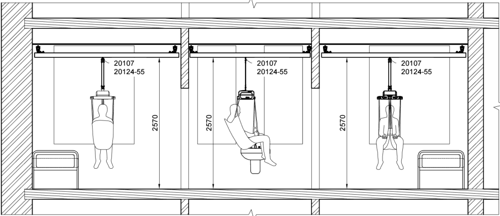
ŘEZ A-A
