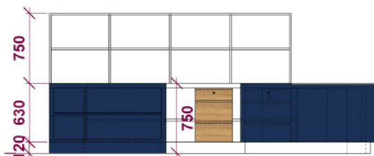
PŮDORYS
