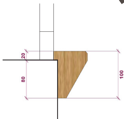
POHLED
