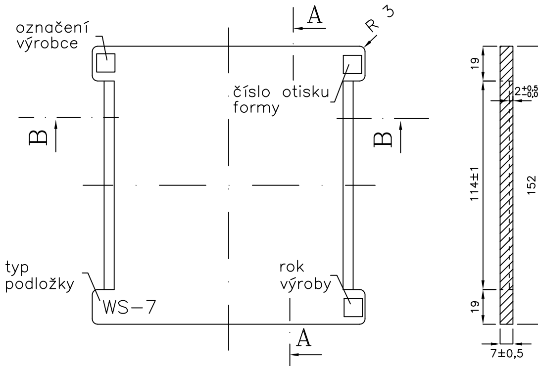
Obraz 2. Řez B – B
