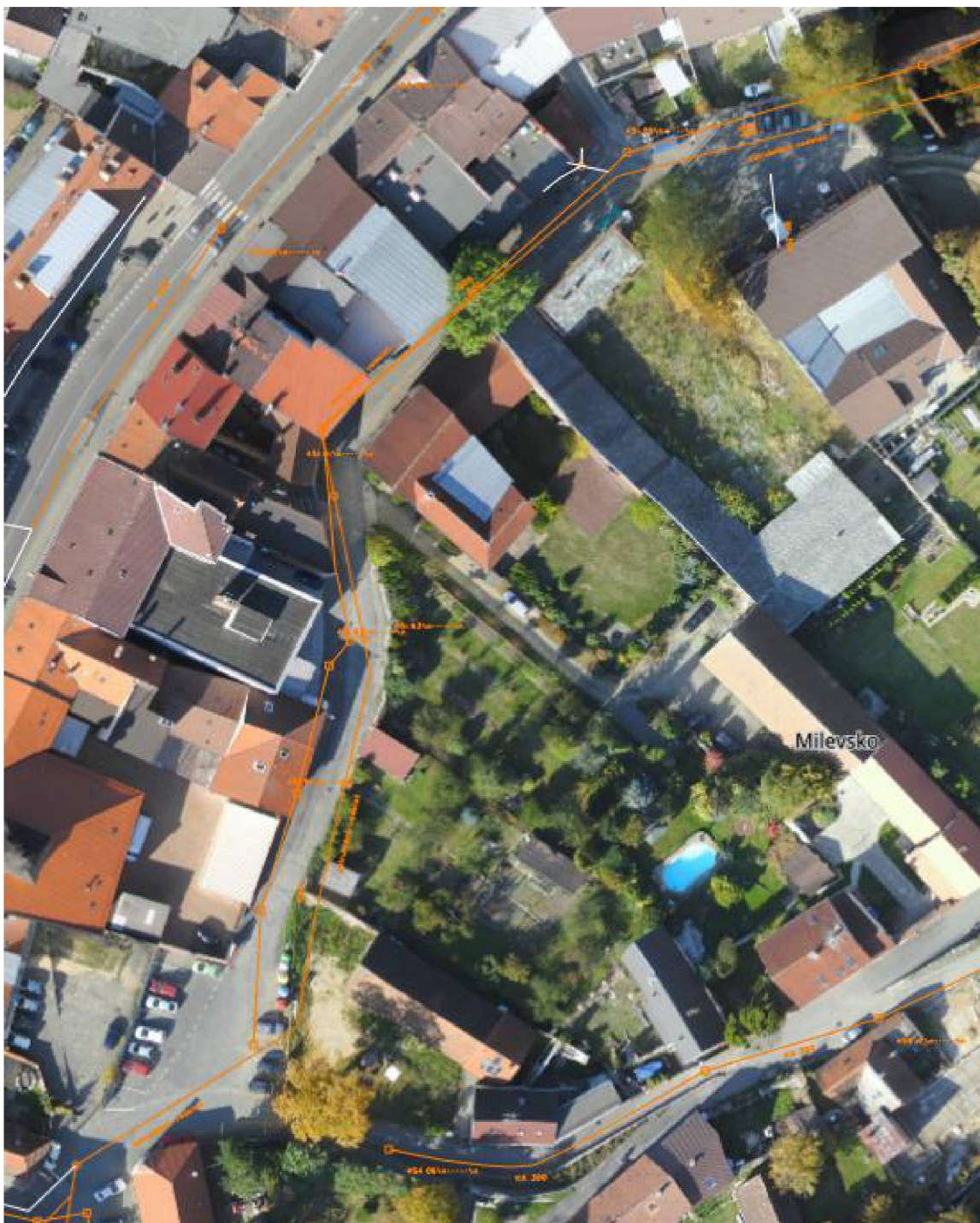
Obr. 2 - Stávající kanalizace a vodoteč
