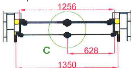
ŘEZ - PŮDORYS
