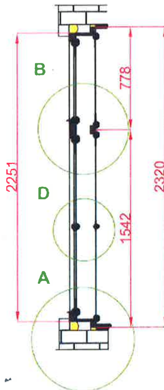
ŘEZ - BOKORYS
