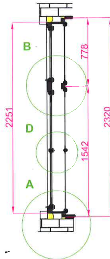
ŘEZ - BOKORYS
