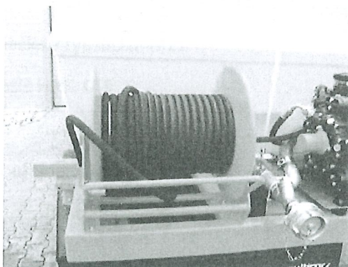
Zadní navíjecí buben s vysokotlakou hadicí
