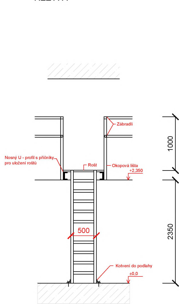
ŘEZ A-A'
